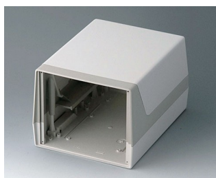
A9917837 LUX CASE 230, исп. I АБС (UL 94 HB) белый RAL 9002 173x230x136mm
