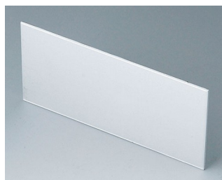
A9199151 Лицевая панель 190 Алюминий матово-анодированный 134x62,5x1,5mm
