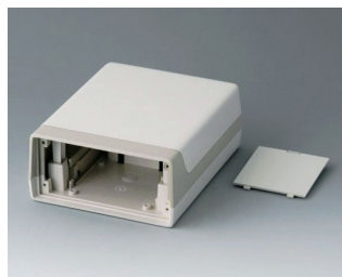
A9912687 LUX CASE 150, исп. II АБС (UL 94 HB) белый RAL 9002 118x150x57mm
