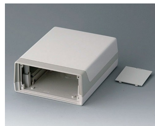
A9915787 LUX CASE 190, исп. II АБС (UL 94 HB) белый RAL 9002 148x190x67mm
